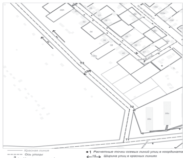
Разбивочный чертёж красных линий в кварталах № 475; 673; 408
